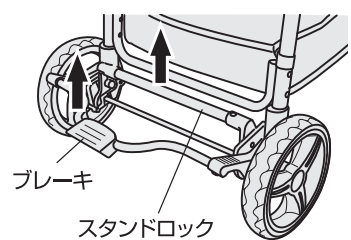
3.スタンドロックを持ち上げて赤色が見えないことを確認し、ブレーキを持ち上げる。
